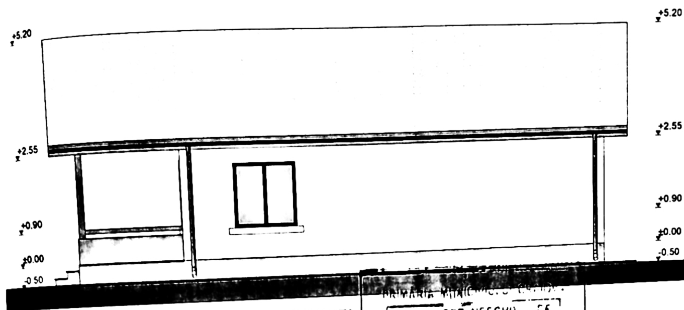
FATADA LATERALA DREAPTA
